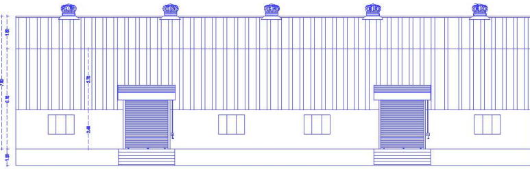
ELEVATION
